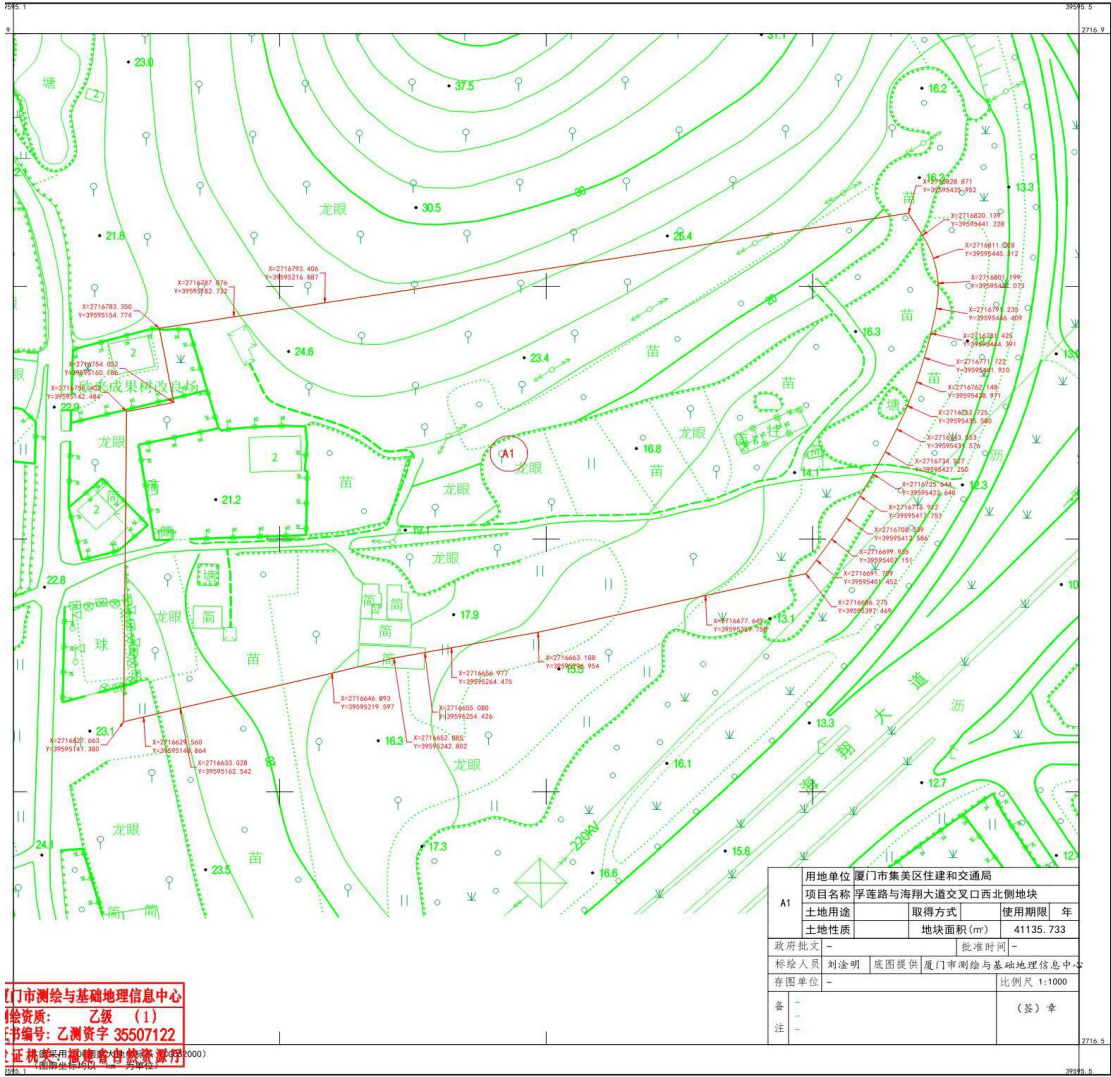
孚莲路与海翔大道交叉口西北侧地块勘测定界图
