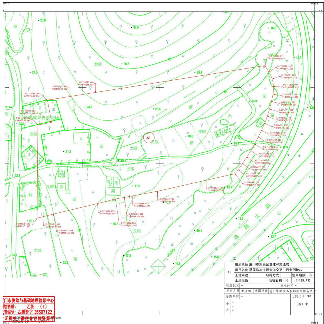
孚莲路与海翔大道交叉口西北侧地块勘测定界图
